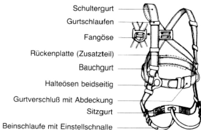
Bild 8: Auffanggurt mit rückseitiger Fangöse und seitlichen Halteösen
