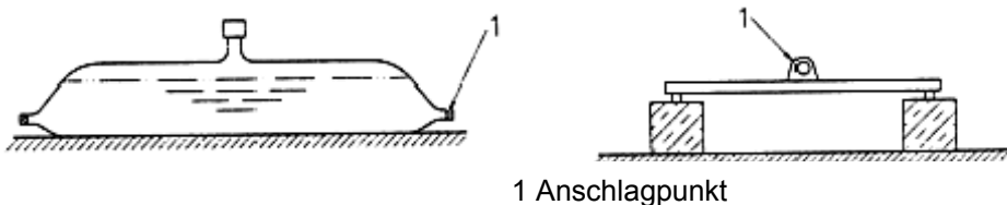
Bild 25: Beispiele für durch Eigengewicht gehaltene Anschlageinrichtungen
