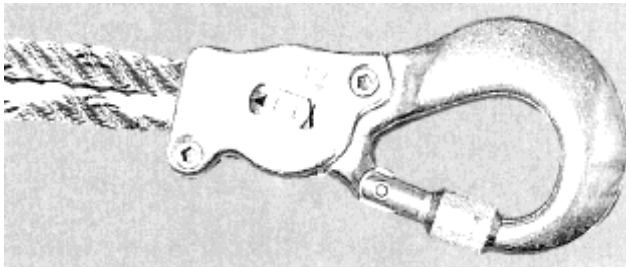
Bild 12: Reibungs-Falldämpfer mit Verbindungsmittel. Der Falldämpfer ist in einem Karabinerhaken integriert
