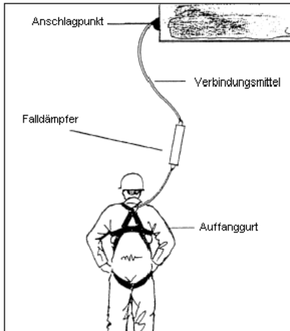
Bild 6: Skizze des Auffangsystems mit Falldämpfer
