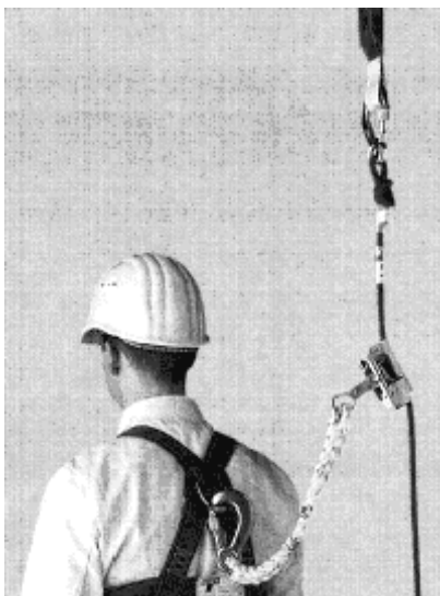
Bild 2: Beispiel des Auffangsystems: Mitlaufendes Auffanggerät einschließlich beweglicher Führung; hier befindet sich der Falldämpfer zwischen der beweglichen Führung und dem Anschlagpunkt
