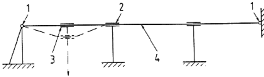
a) Anschlageinrichtung, z.B. auf einem Dach
