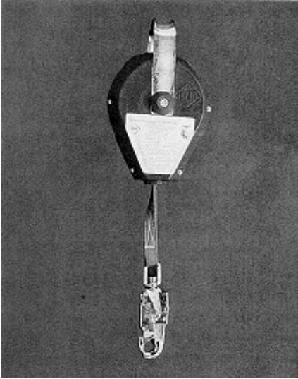
Bild 14: Höhensicherungsgerät mit einziehbarem Verbindungsmittel aus Gurtband
