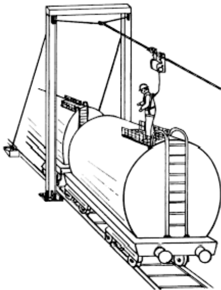
Bild 23: Anschlagkonstruktion kombiniert mit rollbarem Abseilgerät zur Befestigung von persönlichen Schutzausrüstungen gegen Absturz für Versicherte, die auf Kesselwagen unter Absturzgefahr tätig sind
