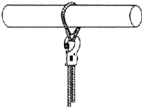
Bild 26: Richtiges Anschlagen: Zur Erhaltung der Funktionsfähigkeit des Falldämpfers wird ein Anschlagverbindungsmittel mit zwei Augen verwendet, welches über ein waagrechtes Tragelement gelegt wird; Einhaken des Karabinerhakens in die zwei Augen
