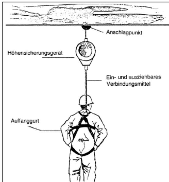
Bild 4: Skizze des Auffangsystems mit Höhsicherungsgerät
